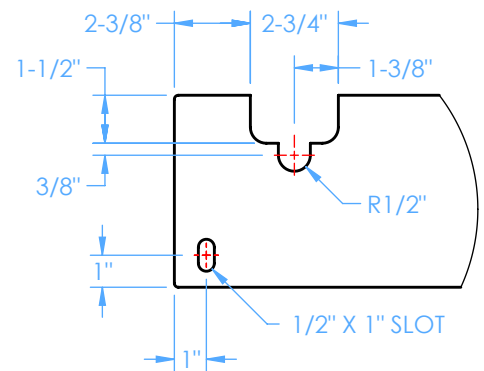
DETAIL A TYP
